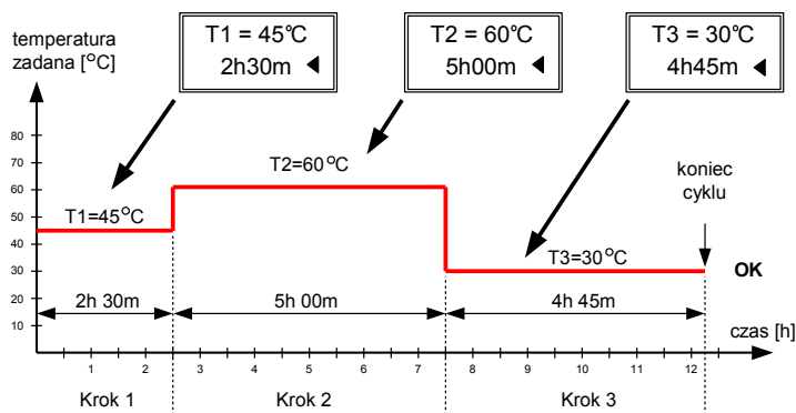
Rys.1 Przykładowy cykl grzania: T1=45°C,2h30m -> T2=60°C,5h00m -> T3=30°C,4h45m.
