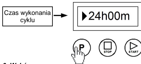
Rys. 3 Wybór programu.
