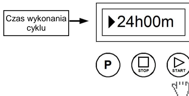
Rys. 4 Uruchomienie programu
